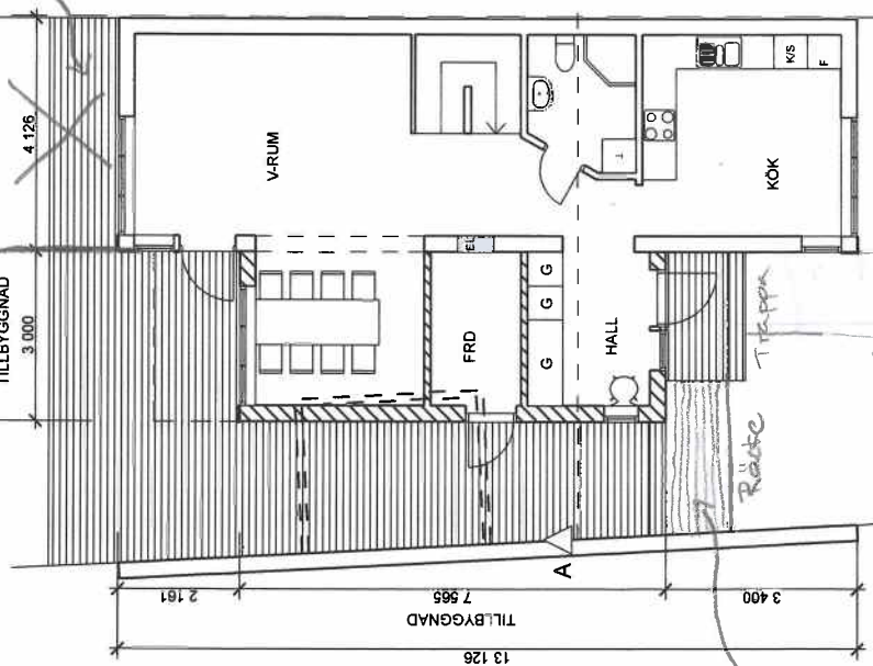
PLAN BOTTENVÅNING 1:100
