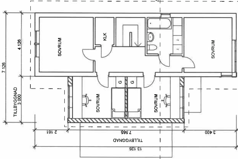
PLAN ÖVERVÄNING 1:100
