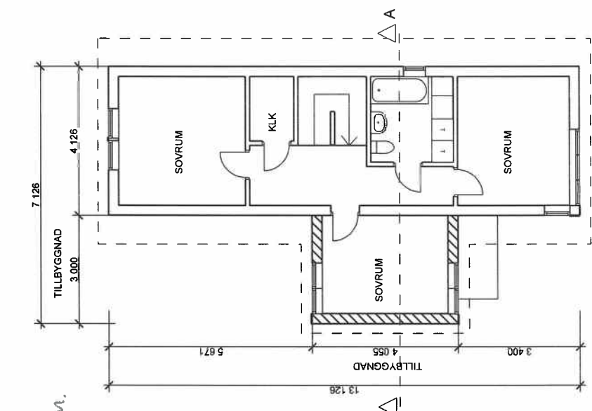
PLAN ÖVERVÄNING
