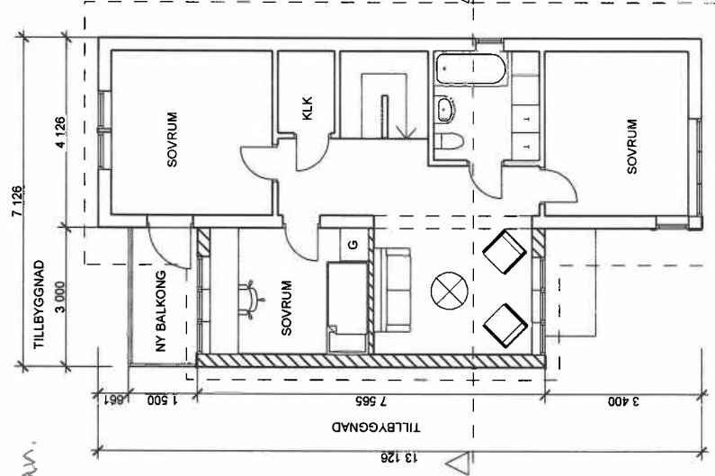
PLAN ÖVERVÅNING 1:100
