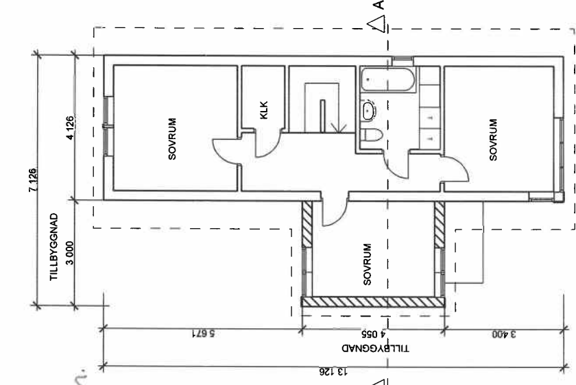
PLAN ÖVERVÄNING
